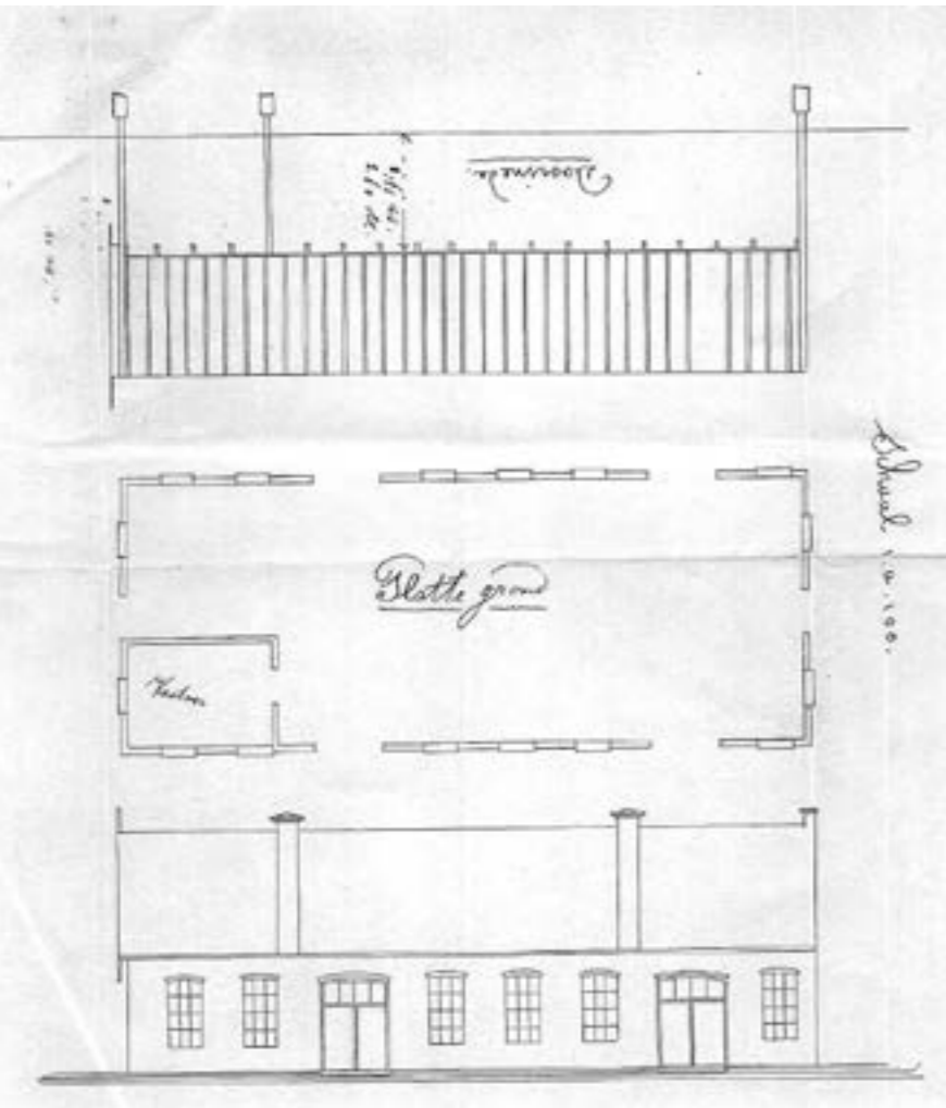
Tekening gebouw cementsteenfabriek Erica (Bron: Gemeente-archief Emmen, hinderwetvergunning 19-9-1905 nr. 41)
