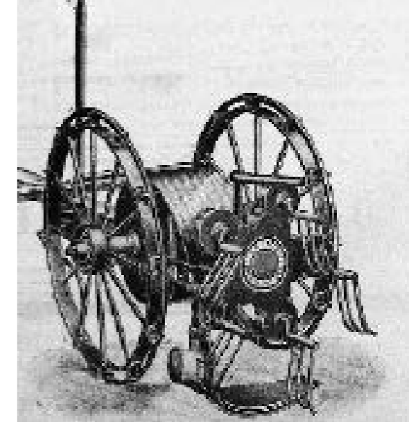
Foto's uit een advertentie uit de Emmer Courant van 30 augustus 1913. Het betrof hier een vergelijking tussen een nieuwe en een oude aardappelrooimachine van de firma Gebr. Kemper, zoals die ook bij landbouwers in Nieuw-Amsterdam en Oranjedorp op dat moment werden gebruikt en die door de boeren werden ingezet wanneer de aardappelkrabbers staakten voor een hogere beloning. Tijdens de Eerste Wereldoorlog kreeg deze firma uit Winschoten ook een filiaal voor de verkoop van landbouwwerktuigen in het dorp Em-
