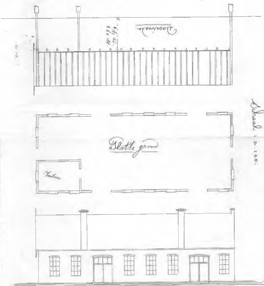
Tekening gebouw cementsteenfabriek Erica (Bron: Gemeente-archief Emmen, hinderwetvergunning 19-9-1905 nr. 41)
