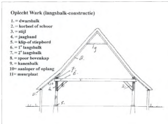
Bouwkundige benamingen 'oplecht warck'. Tekening gemaakt door Auke Radelaar.
