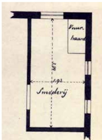
Bouwtekening van de rijwielherstelplaats van Houwinus Thedinga met de afmetingen van 1,93m bij 3,84m - in het pand van Hilbrands.
